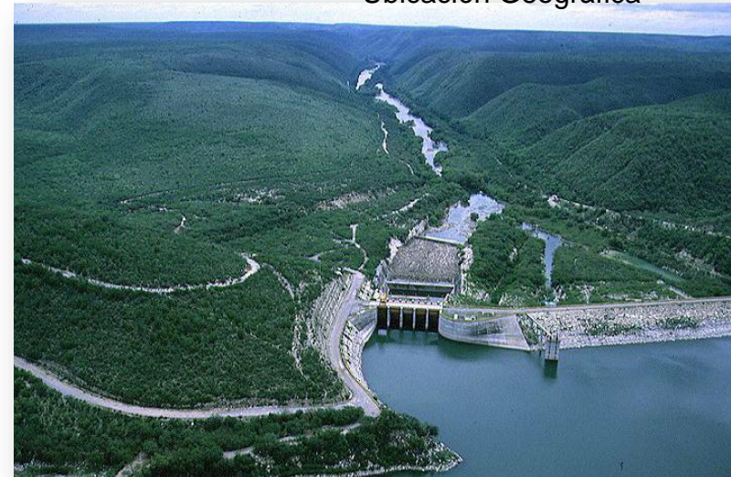
Vertedor Presa General Vicente Guerrero CIN.
